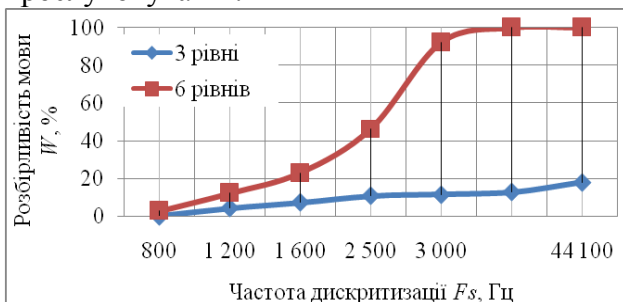
Рисунок 3 – Залежність розбірливості мови W від частоти дискретизації F_s при різній кількості рівнів квантування
