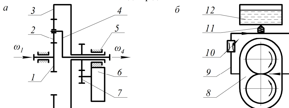
Рис. 1. Схеми: а – зубчастої диференціальної передачі з керуванням через епіцикл та ведучою ланкою – сонячним зубчастим колесом; б – замкнутої гідросистеми
