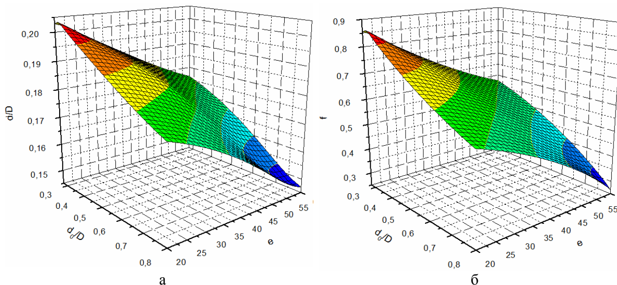
Рис. 1. Степень (а) и интенсивность (б) заковки отверстия при ковке полых цилиндров бойками с углом выреза \alpha = 115^\circ и подачами 0,1D
