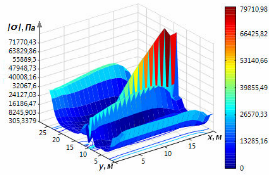
Рисунок 11. Графік розподілу поля модуля напружень із урахуванням тепло-масоперенесення
