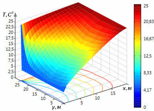
Рисунок 6. Графік розподілу поля температури при фільтрації сольових розчинів
