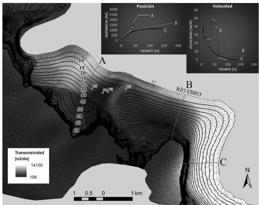
Fig. 4.- Mapa de isócronas del frente de propagación de la recarga para el acuífero aluvial y evolución de la velocidad de la recarga. Las líneas A, B y C representan tres trayectorias del frente de propagación.
