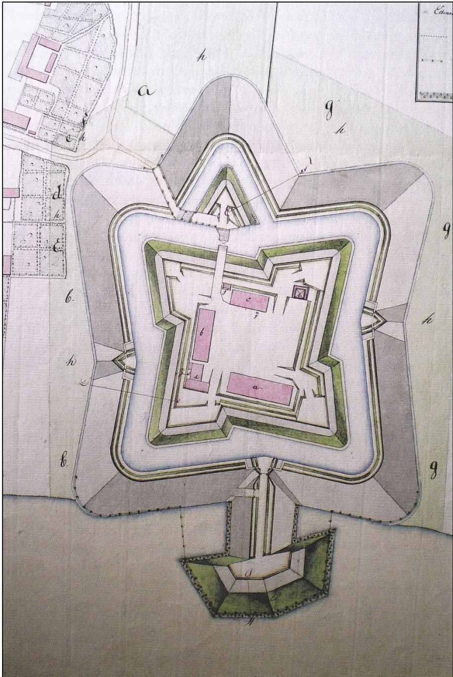
Fig. 11. Opmåling af Hals Skanse 1801. Signaturerne i skansegården angiver følgende: a. Grundmuret barak. b. Nybygget barak af bindingsværk beklædt med
