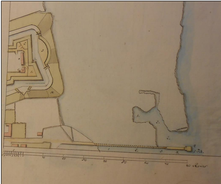
Fig 9. Situationsplan, Hals Skanse, sydlige del, 1798. 989 Nord er til venstre. Nr. 1 og 2 angiver batterierne på sydvolden, mod øst og vest, og nr. 3 det projekterede søbatteri, eller batterie á fleur d'eau. Bygning a er den sydlige, grundmurede kommandantbolig og barak, b er kostald og materielhus, c er svinesti og d er vandhus, dvs. et lokum i voldgraven, hvortil fører en tunnel gennem sydvolden. Efter som situationsplanen er udarbejdet ifm. det projekterede søbatteri, er kun de sydlige bygninger i skansen angivet. Til gengæld ses Hals skibsbro nederst i billedet, og over den Hals havn, som man i 1799 overvejede at tage i brug som flådehavn.
