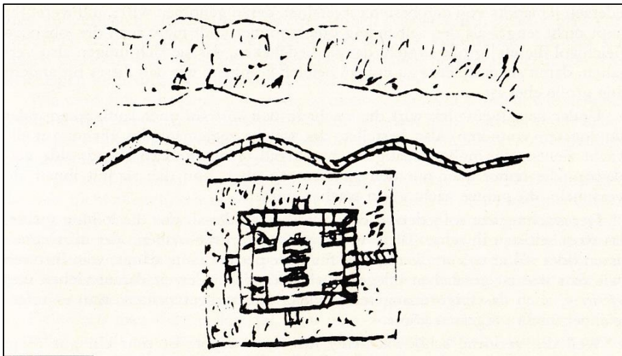
Fig. 3. Redoute i grev Johann von Nassau-Siegens krigsbog 1597-1623. Redouten kan i denne udformning opfattes som idealtype, og har været beregnet til minimum fire kanoner. 159
