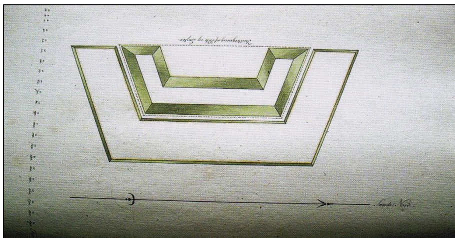
Fig 13. Epaulement for kavaleri ved Egense 1810. 1060
