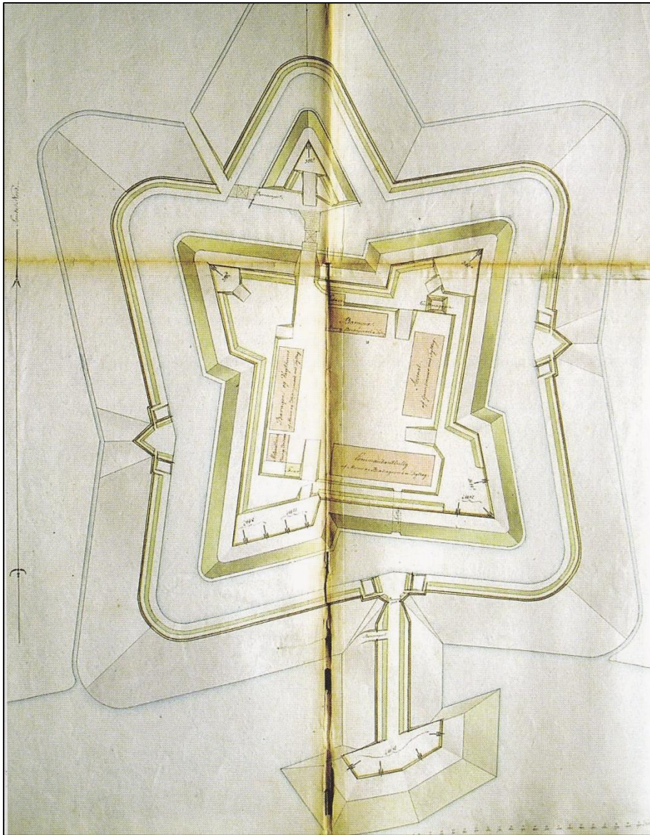
Fig. 15. Hals Skanse 1810. Bemærk at der er angivet tunnel i sydvolden og en bygning ved østvolden. Det drejer sig om det endnu eksisterende Tøjhus, der sammen med krudtkammeret nord for dette er de eneste bevarede bygninger i skansen. 1067
