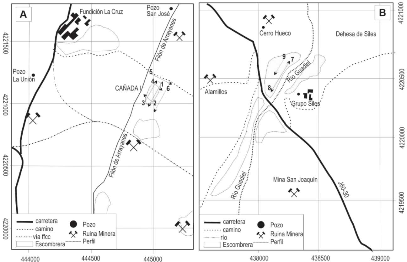
Fig. 2.- Localización de los radargramas realizados (1-9). A) Afloramiento de La Mejor 1ª-2ª. B) Afloramiento de La Cañada I. Fig. 2.- Radargrames location (1-9). A) La Mejor 1ª-2ª outcrop. B) La Cañada I outcrop.
