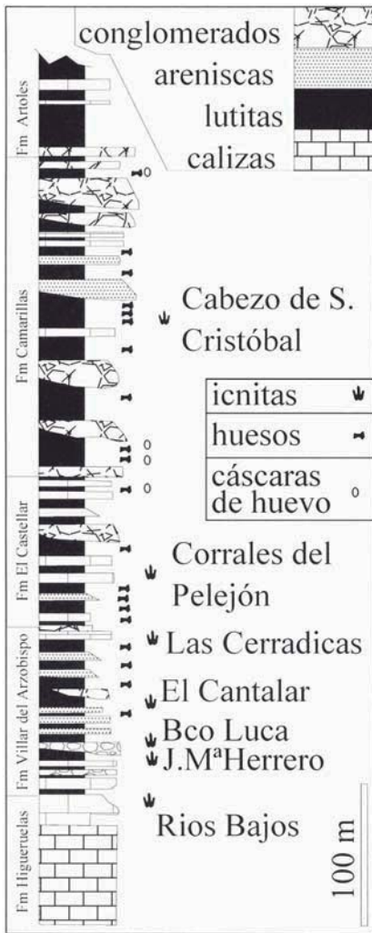
Fig. 2.- Serie estratigráfica (Jurásico Superior-Cretácico Inferior) de Galve. Situación de los yacimientos de restos directos e indirectos de dinosaurios. Modified from Ruiz Omeñaca et al. (2004).
