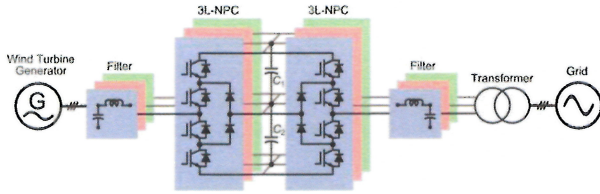
Fig. 9. 3L-NPC BTB topology for WTSs.
