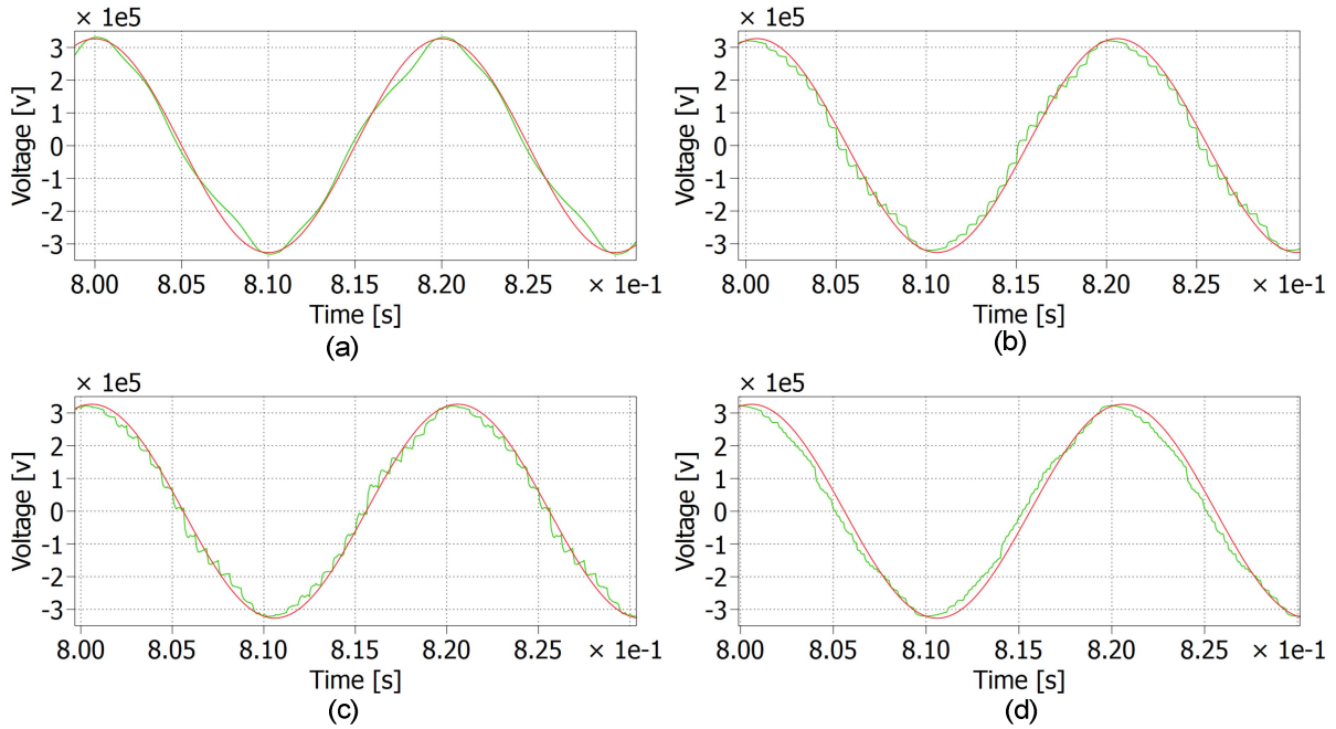
Fig. 7 Output voltage: (a) PSC-PWM (b) NLC (c) NLC+PWM (d) NLC+CRG.
