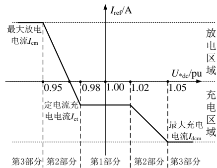
(b) 下垂环节特性
