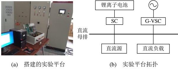
图 13 实验平台
