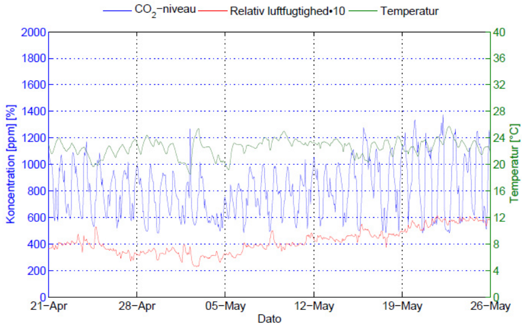
Figur 46. Målinger af indetemperatur, CO 2 og relativ fugtighed i opholdsstuen i perioden 21.4.2014 - 26.5.2014, efter montering af Energy Frames. For hele perioden ligger gennemsnitstemperaturen omkring 23 °C. Figur 46 viser, at temperaturerne i alle huset rum generelt ligger lidt lavere end i perioden før monteringen af de isolerende skodder. Udetemperaturen svingede kraftigt i perioden, med en middelværdi på ca. 14 °C, se figur 47, dvs. den lå betydeligt højere end i den første periode.
