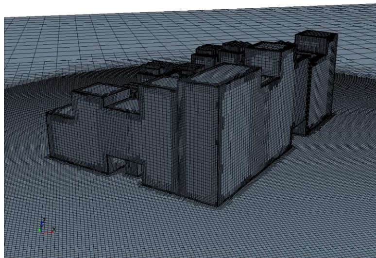
Figur 2.2 Beregningsnet omkring den nye geometri af kanalhusene
