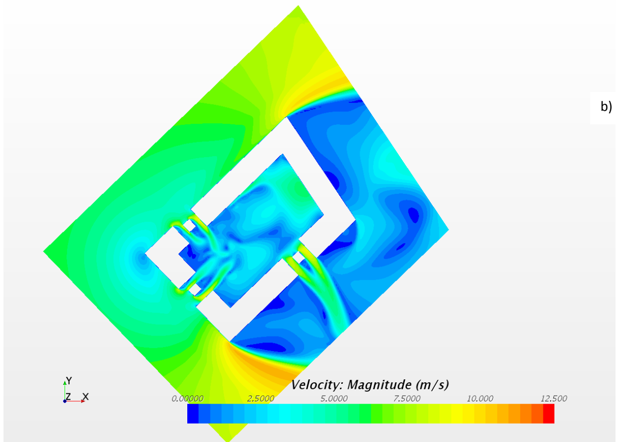
Figur 4.4 Vindhastigheder ved vindretning 270 (østlig vind) for a) oprindelig geometri og b) ny geometri
