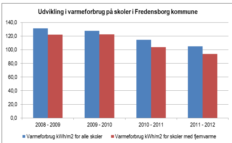
Figur 16. Udvikling i varmekonsum på skolerne i Fredensborg kommune
