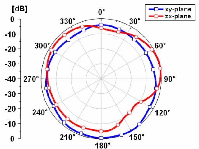
(d) Radiation pattern at 1920MHz.
