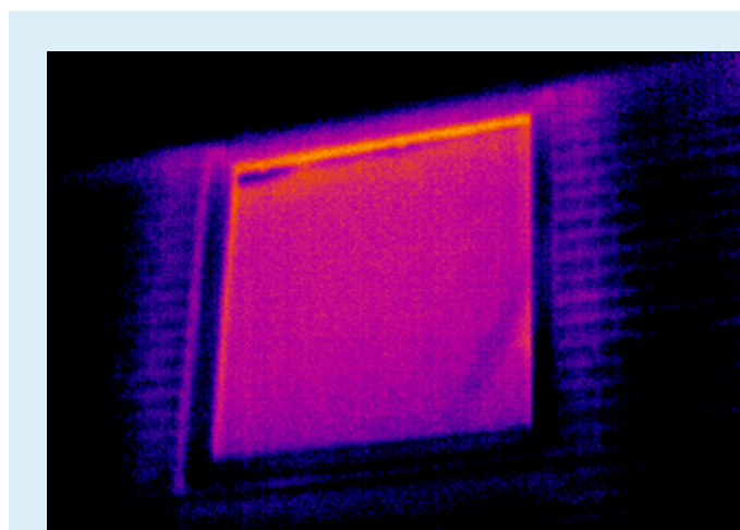
Termografisk billede af samling ved vindue.
