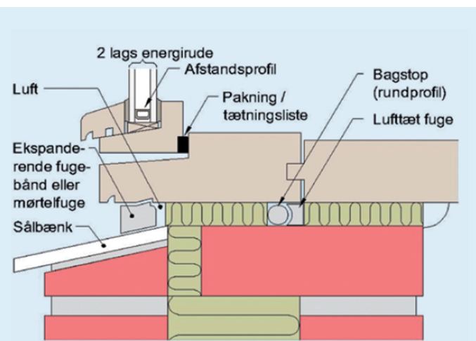
Vinduesfals med kuldebroisolering mellem for- og bagmur.
