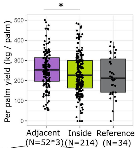
a) Per palm yield
