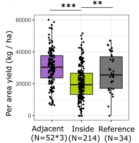
b) Per area yield
