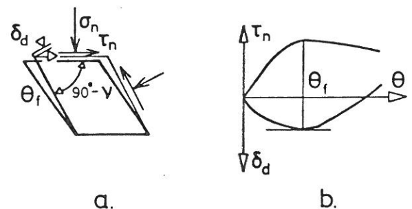
Fig. 8 Pure shear
