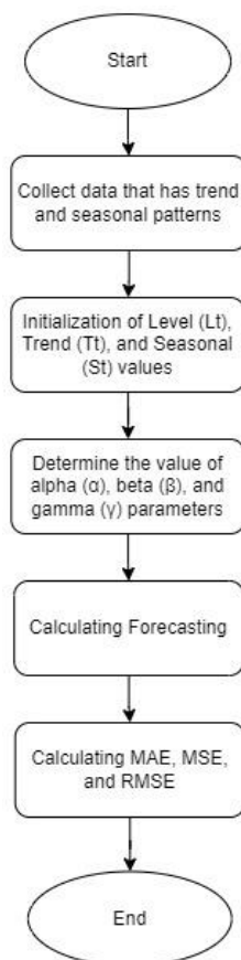
Gambar 3 Tahapan Metode HWES
