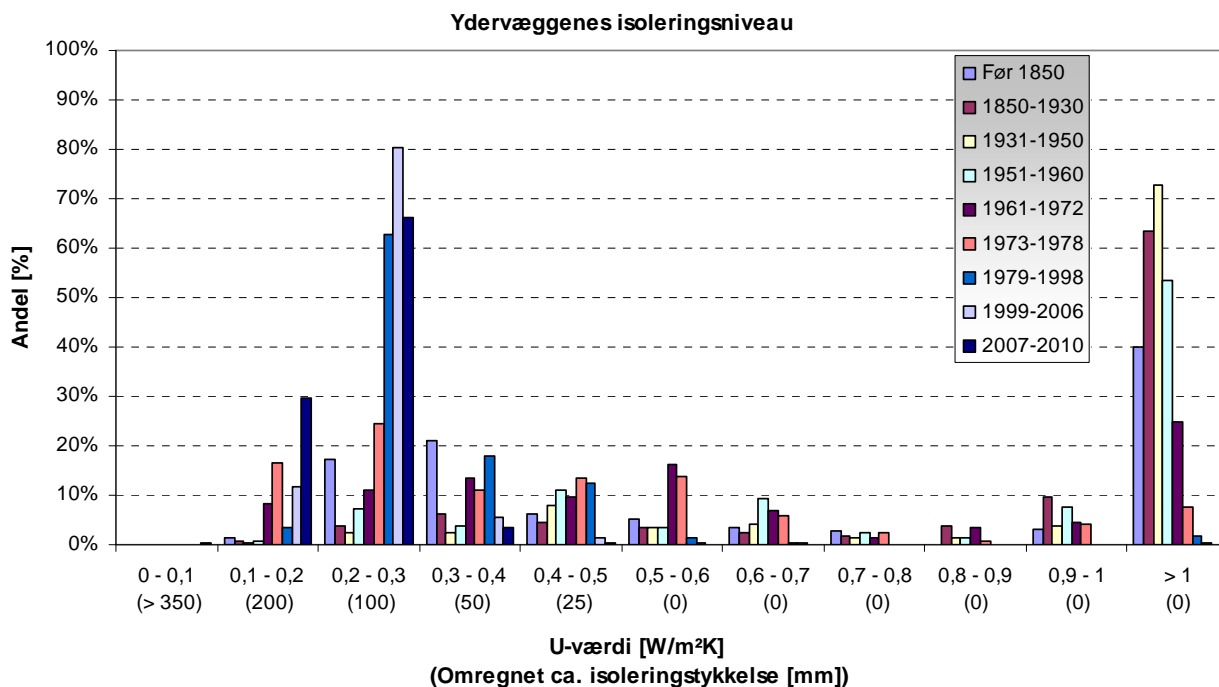
Figur 3 Lofternes isoleringsniveau er fundet ved en arealvægtning af samtlige registrerede U-værdier for konstruktioner med sfb kode 31 (Ydervægge). U-værdierne er omregnet til en tilsvarende ca. isoleringstykkelse med antagelse af en standard tung ydervægskonstruktion.
