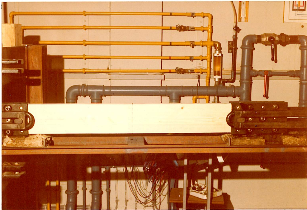
Figur 3. Prøvelegeme med påmonterede stållaskebeslag til overføring af prøvelasten (træk). Kraften overføres fra prøvemaskinens belastningsarrangement gennem de viste stænger. Disse er vandkølede for at hindre indbrænding i træet mellem stållaskerne. Efter monteringen skydes hele det viste arrangement sideværts ind i brandkammeret.
