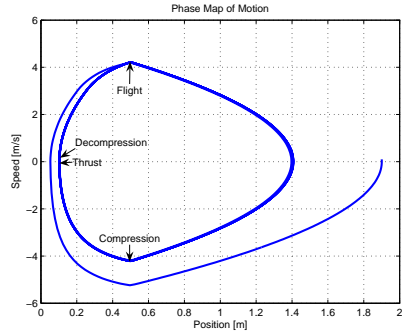
(d) Phase-plane portrait
