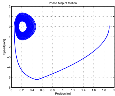
(d) Phase-plane portrait
