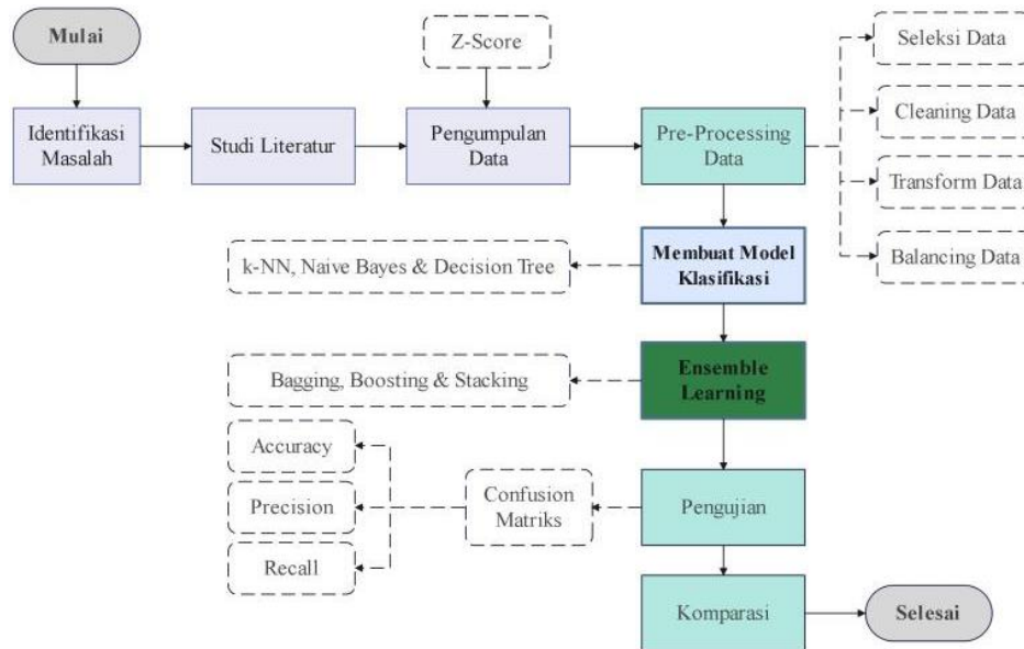
Gambar 1 Tahapan Penelitian
