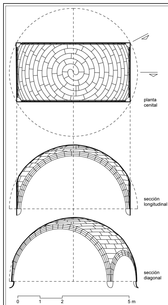
Fig. 2. Planta y secciones de la bóveda baída.
