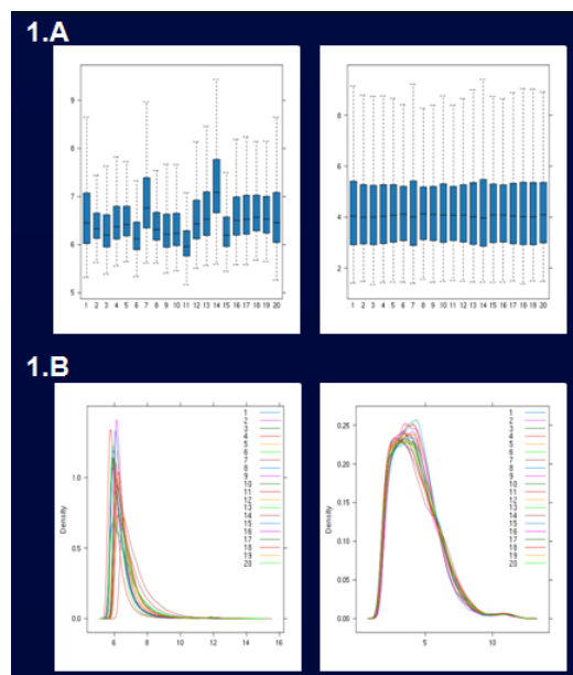
Figura 1. 1.A). Diagrama de cajas del log2 (Intensidades). Cada caja se corresponde con un array. Podemos comprobar que tras la normalización los microarrays son homogéneos ya que las cajas son de amplitud similar y están centradas en posiciones cercanas de el eje Y; Figura 1.B). Representación gráfica de la calidad del material biológico, en este caso ARN, empleado. Cada línea de corresponde con una muestra hibridada en un microarray.
