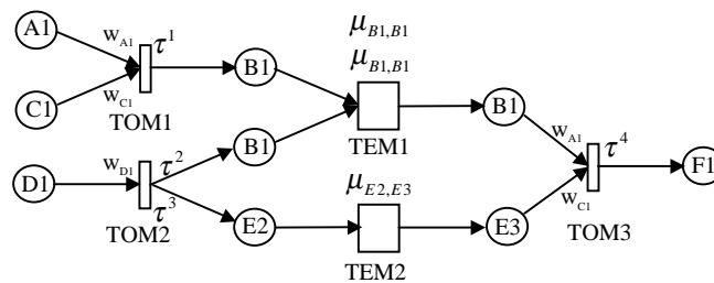
Fig. 1. Estructura gráfica general de una base de reglas en el formalismo hardware-FPN
