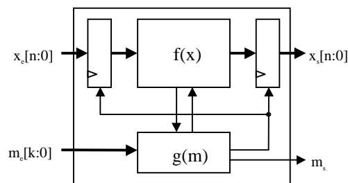
Fig. 2. Estructura general de los módulos del formalismo hardware-FPN
