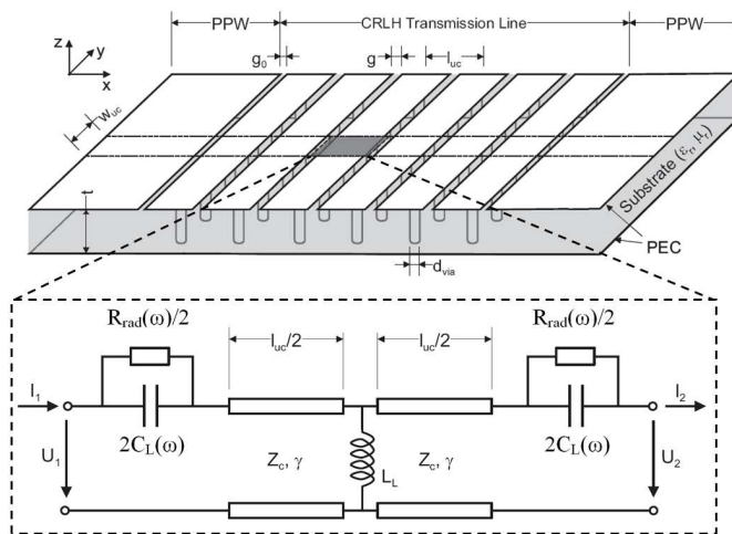
Fig. 1: Esquema de una antenna CRLH PPW leaky-wave, alimentada por dos guías de onda. En la parte inferior, se observa el modelo equivalente dispersivo de una celda unidad.
