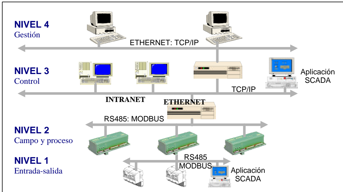
Figura 1: Sistema global de comunicaciones (modelo CIM)
