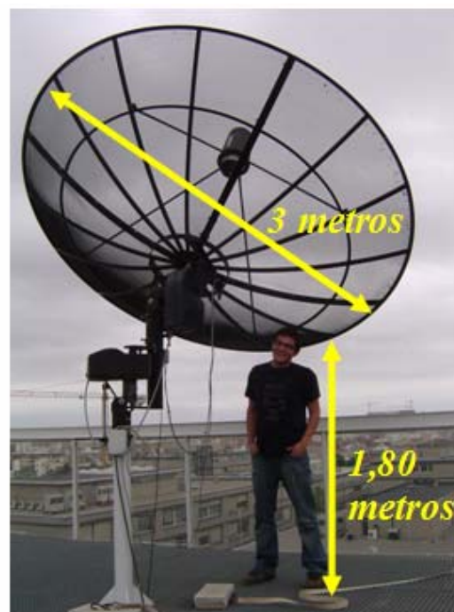
b) Antena del Radiotelescopio de la UPCT
