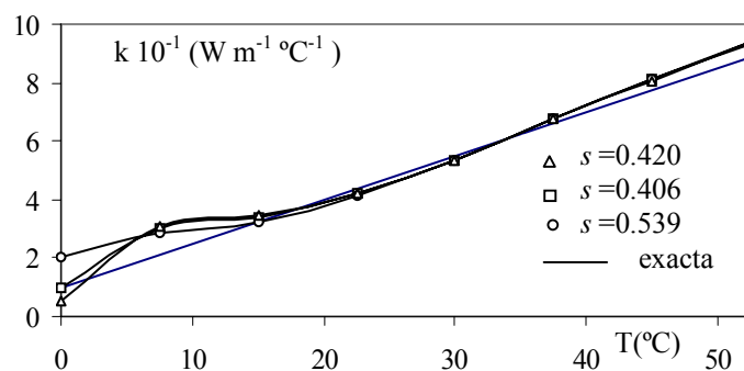
Figura VII.44. Estimación de la conductividad térmica para el caso lineal, en función de varios puntos iniciales, \Delta T_a = 15 \text{ °C} , x_f=0
