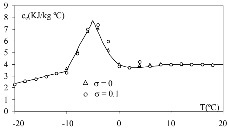
Figura VII.33. Estimación del calor específico, para \sigma = 0 y \sigma = 0.1
