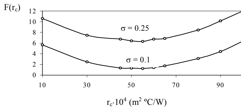
Figura VI.13. Curva de sensibilidad F(r_c) , \sigma = 0.1 y 0.25 , h = 100 Wm^{-2} \text{ } ^\circ C^{-1} , \Delta t = 15 s
