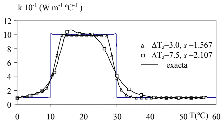
Figura VII.55. Punto de medida en la superficie adiabática, \Delta T_a = 3 y 7.5\text{ °C}
