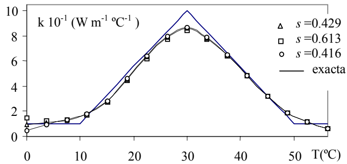
Figura VII.48. Estimación de la conductividad térmica para la dependencia triangular, en función del punto inicial, \Delta T_a=7.5^\circ\text{C} , x_f=0
