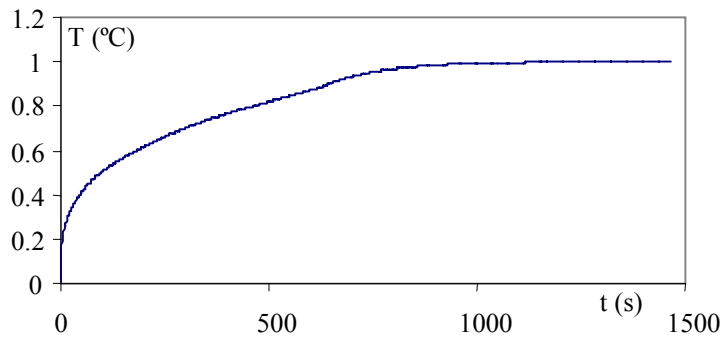
Figura VII.19. Solución del problema directo, T(x_f=L,t) . Dependencia rectangular
