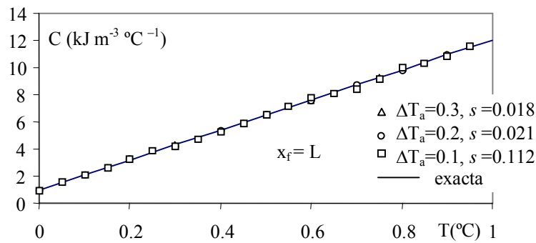
Figura VII.6. Influencia de \Delta T_a en la estimación de la capacidad calorífica para dependencia lineal. c_e = 1+11T , sin error, \Delta T_a = 0.2 y 0.3 °C, \Delta t = 0.1 s
