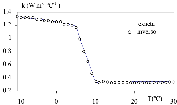
Figura VII.65. Conductividad térmica de las fresas, \sigma=0 , \Delta T_a=2^\circ\text{C} y \Delta t=5 s
