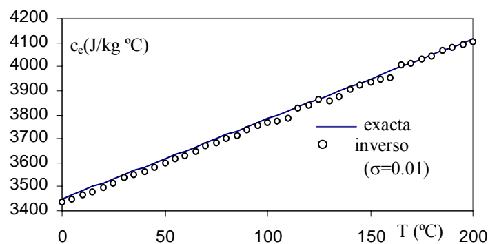
Figura VII.66. Calor específico del hierro, \sigma=0.01 , \Delta T_a=2^\circ\text{C} y \Delta t=5 s
