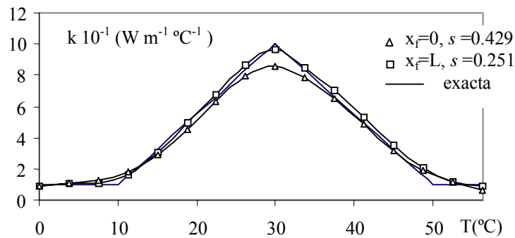
Figura VII.49. Comparación de los distintos extremos de medida, \Delta T_a=7.5^\circ\text{C}
