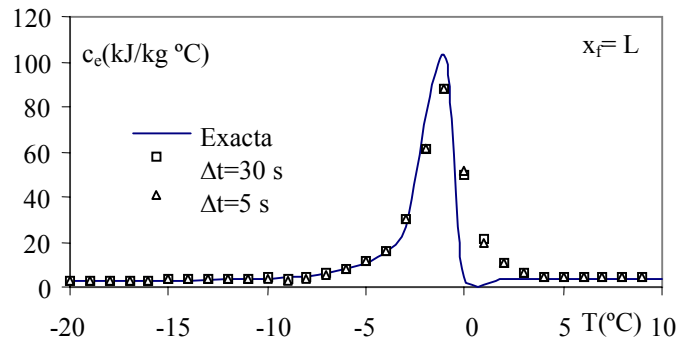
Figura VII.38. Estimación del c_e del pescado blanco. \Delta T_a = 2^\circ\text{C} , \Delta t = 5 y 30 s
