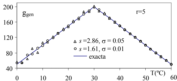
Figura VI.3. Estimación de la generación interna de calor en función de la temperatura del medio
