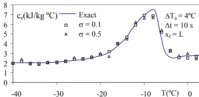
Figura VII.40. Estimación del c_e de la carne de ternera. \Delta T_a = 4^\circ\text{C} , \Delta t = 10 s, \sigma = 0.1 y 0.5
