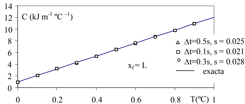
Figura VII.7. Influencia de \Delta t en la estimación de la capacidad calorífica para dependencia lineal. c_e = 1+11T , sin error, \Delta T_a = 0.2 °C, \Delta t = 0.1, 0.3 y 0.5 s
