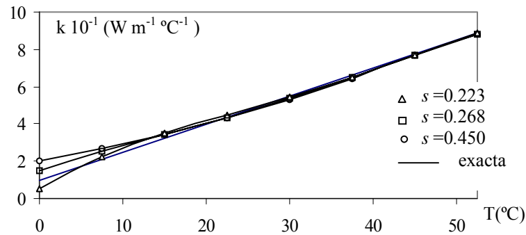
Figura VII.45. Estimación de la conductividad térmica para el caso lineal, en función de varios puntos iniciales, \Delta T_a = 15\text{ °C} , x_f = L
