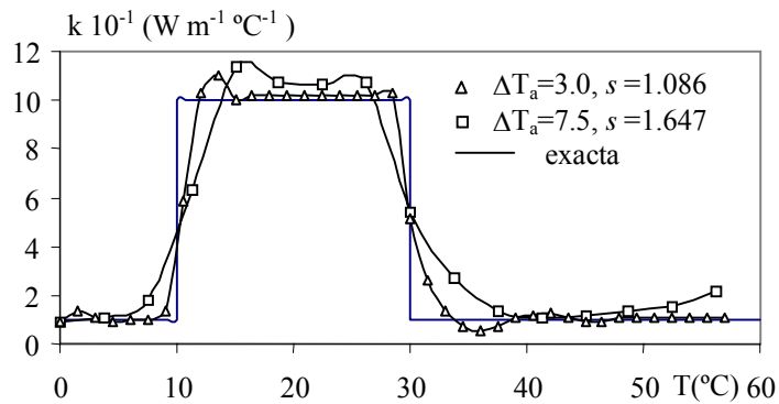
Figura VII.55. Punto de medida en la superficie adiabática, \Delta T_a = 3 y 7.5\text{ °C}
