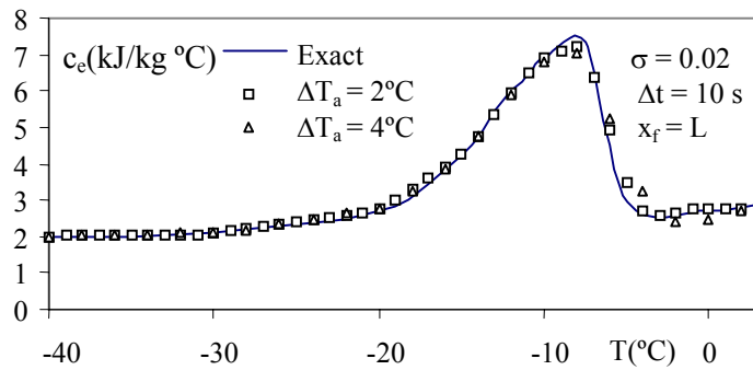
Figura VII.39. Estimación del c_e de la carne de ternera. \Delta T_a = 2 y 4^\circ\text{C} , \Delta t = 10 s, \sigma = 0.02
