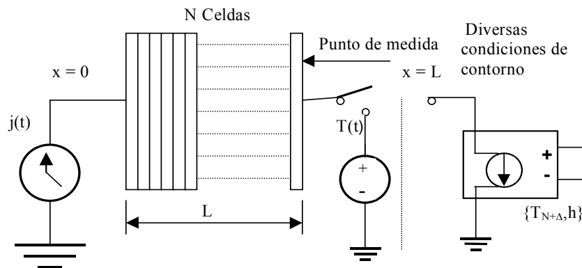
Figura IV.16. Modelo en red para la determinación del flujo de calor incidente
