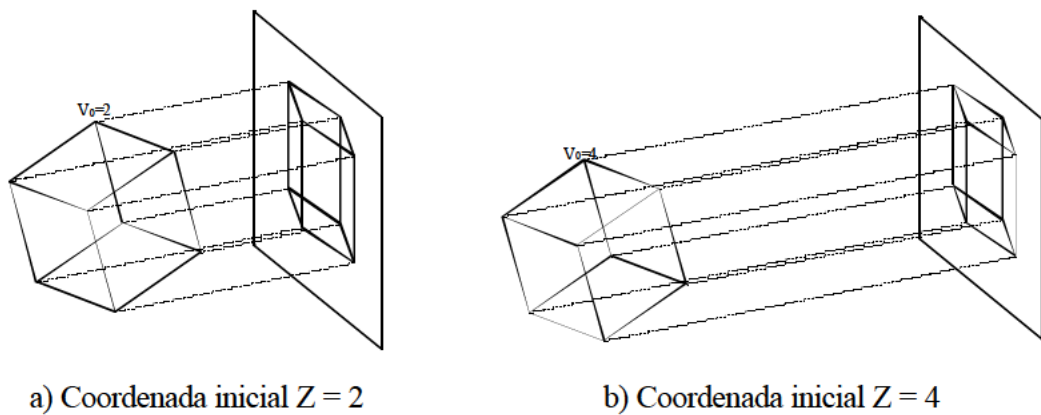
Figura 70. Efectos de la asignación de coordenada inicial arbitraria en el inflado axonométrico
