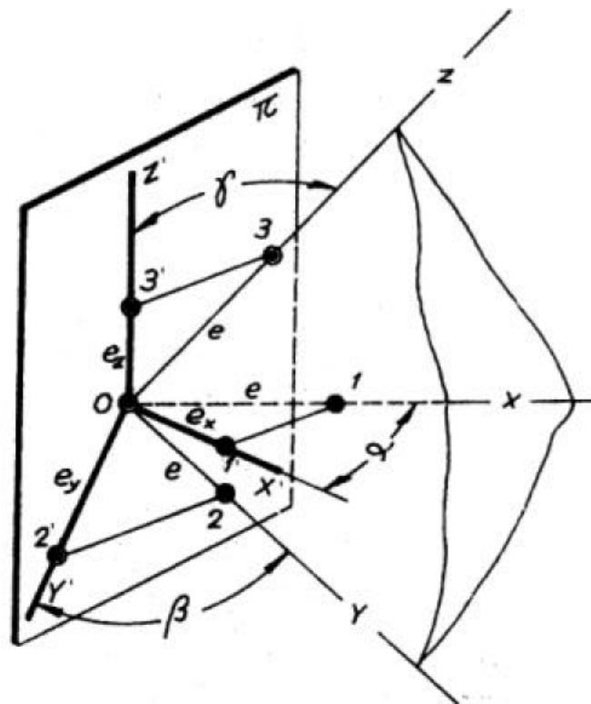
Figura 181. Deducción de los coeficientes de reducción a partir de los ángulos que forman los ejes con sus proyecciones.
