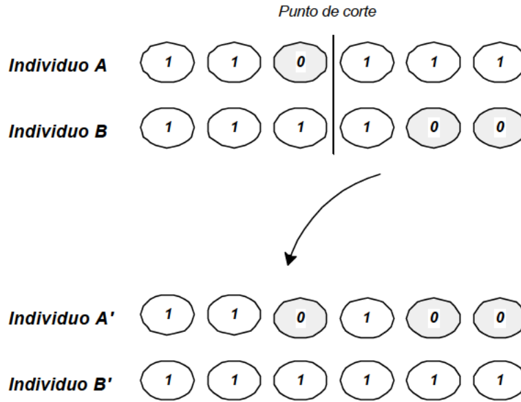
Figura 179. Recombinación de cadenas
