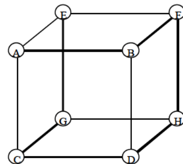
Figura 108. Definición de camino en un grafo
