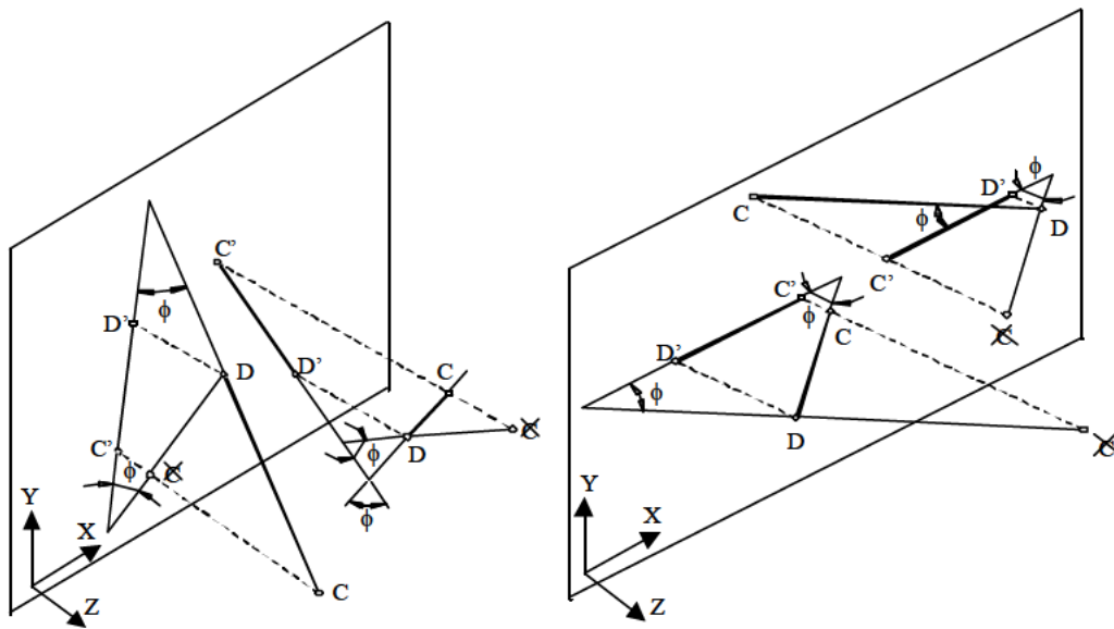
Figura 73. Criterios para la selección en la orientación del ángulo axonometrico
