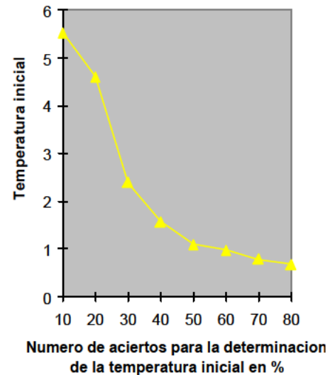
Figura 61. Efectos del coeficiente de aceptación en la determinación de la temperatura inicial
