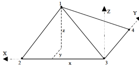
Figura 66. Plano oblicuo en un modelo asimétrico
