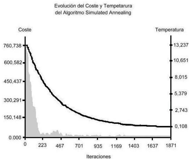
Figura 60. Representación del coste y la temperatura para un paso inicial igual al 4% min (RangoX, RangoY)
