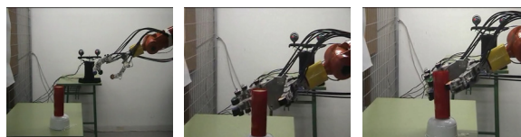
Figura 3. Secuencia de alcance y agarre con el robot antropomorfo PALOMA2
