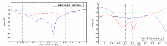
Figura 6. Parámetro S_{11} para los elementos 1 y 3 (izda.) y para los elementos 2 y 4 (dcha.).
