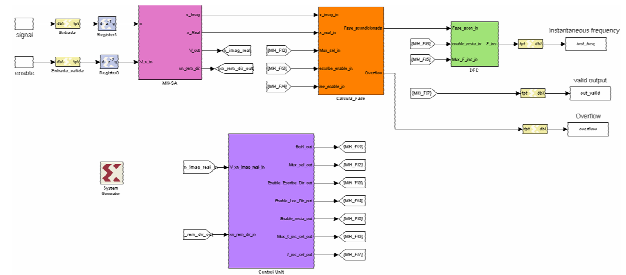
Fig. 2. Diagrama de bloques del cálculo de la FI.
