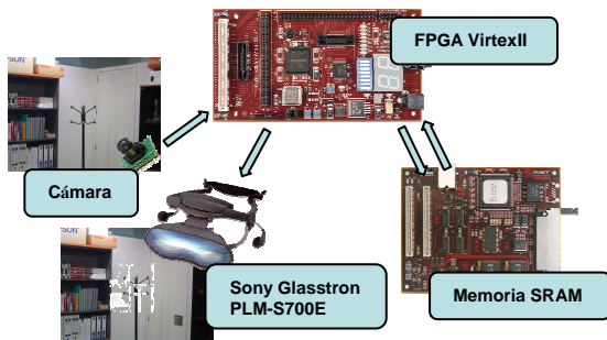
Fig. 1. Estructura a nivel de placas de desarrollo.
