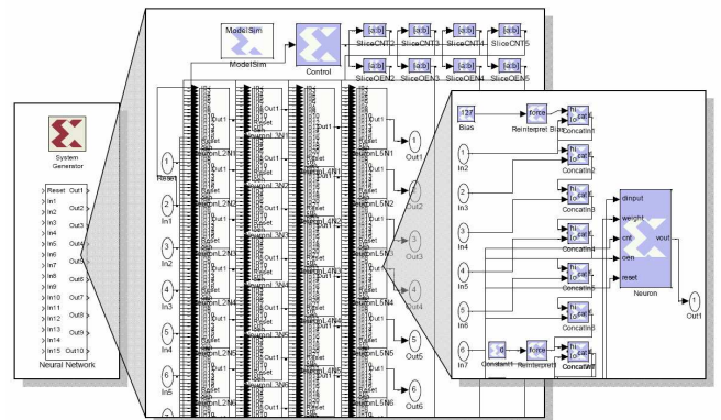
Fig. 3. Vista jerárquica del modelo de un MLP creado por la herramienta, mostrando la estructura de la red.
