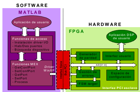
Fig. 4. Estructura de bloques del sistema PCI.
