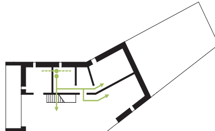
Fig. 3 1. salsplan Ventilation
