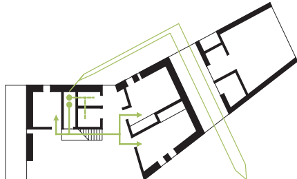
Fig. 2 Stueplan Ventilation Jordvarme
