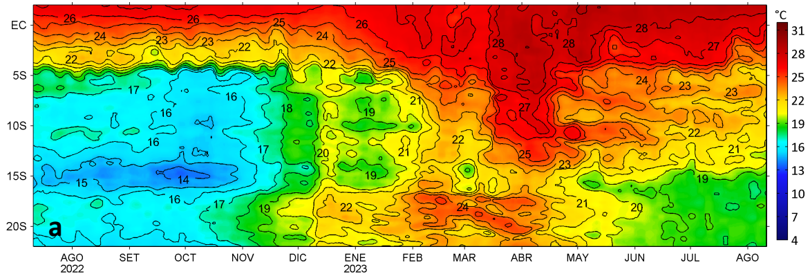
Anomalías de la Temperatura Superficial del mar (°C), franja costera de 60 mn 11 de julio 2022 - 11 de agosto 2023
