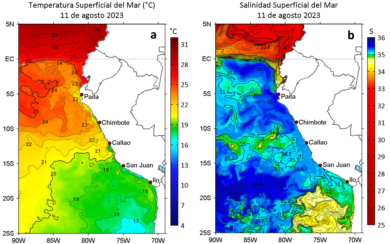
Figura 2. a) Temperatura superficial del mar (°C) y b) Salinidad superficial del mar para el 11 de agosto de 2023. Datos: OSTIA-UKMO-L4-GLOB-v2.0 (UK Met Office, 2012; Donlon et al, 2012) y del GLOBAL_ANALYSISFORECAST_PHY_001_024 (Lellouche, J. M. et al, 2013), respectivamente.
