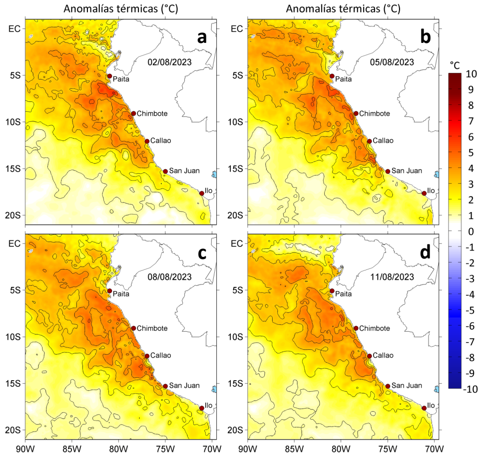
Figura 3. Anomalías de la temperatura superficial del mar (°C) para el a) 02, b) 05, c) 08 y d) 11 de agosto de 2023. Las anomalías se calcularon respecto de la climatología para el periodo 2007-2016. Datos: OSTIA-UKMO-L4-GLOB-v2.0 (UK Met Office, 2012; Donlon et al, 2012).
