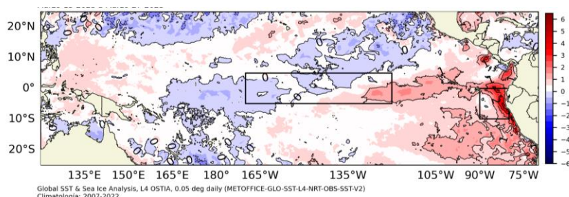
Figura 1: Promedio (del 15 al 27 de marzo) de las anomalías de la TSM en el Pacífico tropical. Las regiones Niño 3.4, en el centro del Pacífico, y Niño 1+2, frente a la costa peruana, están delimitadas con recuadros.
