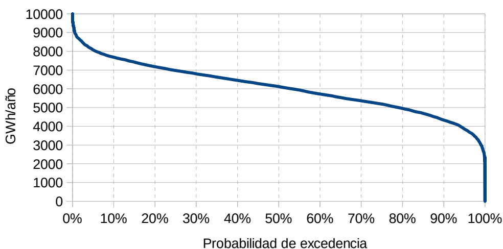
Fig. 1: Variabilidad de la generación hidroeléctrica anual del Uruguay.
