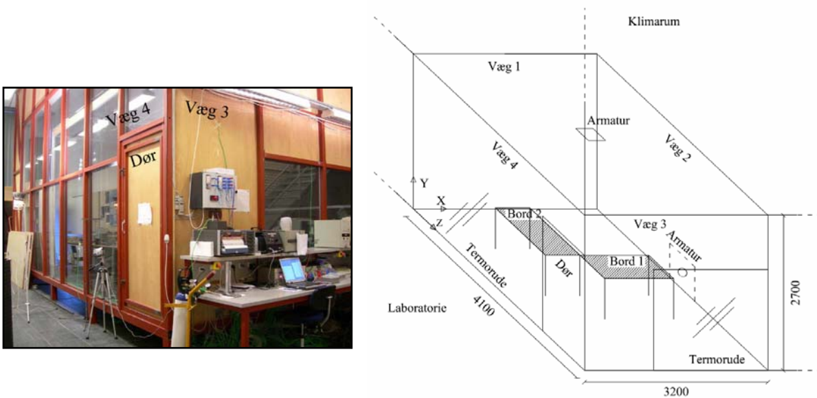
Figur 5. Forsøgsrum hvor der er foretaget eksperimentelle undersøgelser af personbevægelsernes indflydelse på bakterietransport. Forsøget udføres med virkelige personer, mens der dog anvendes sporgas til at simulere bakterier af praktiske grunde.
