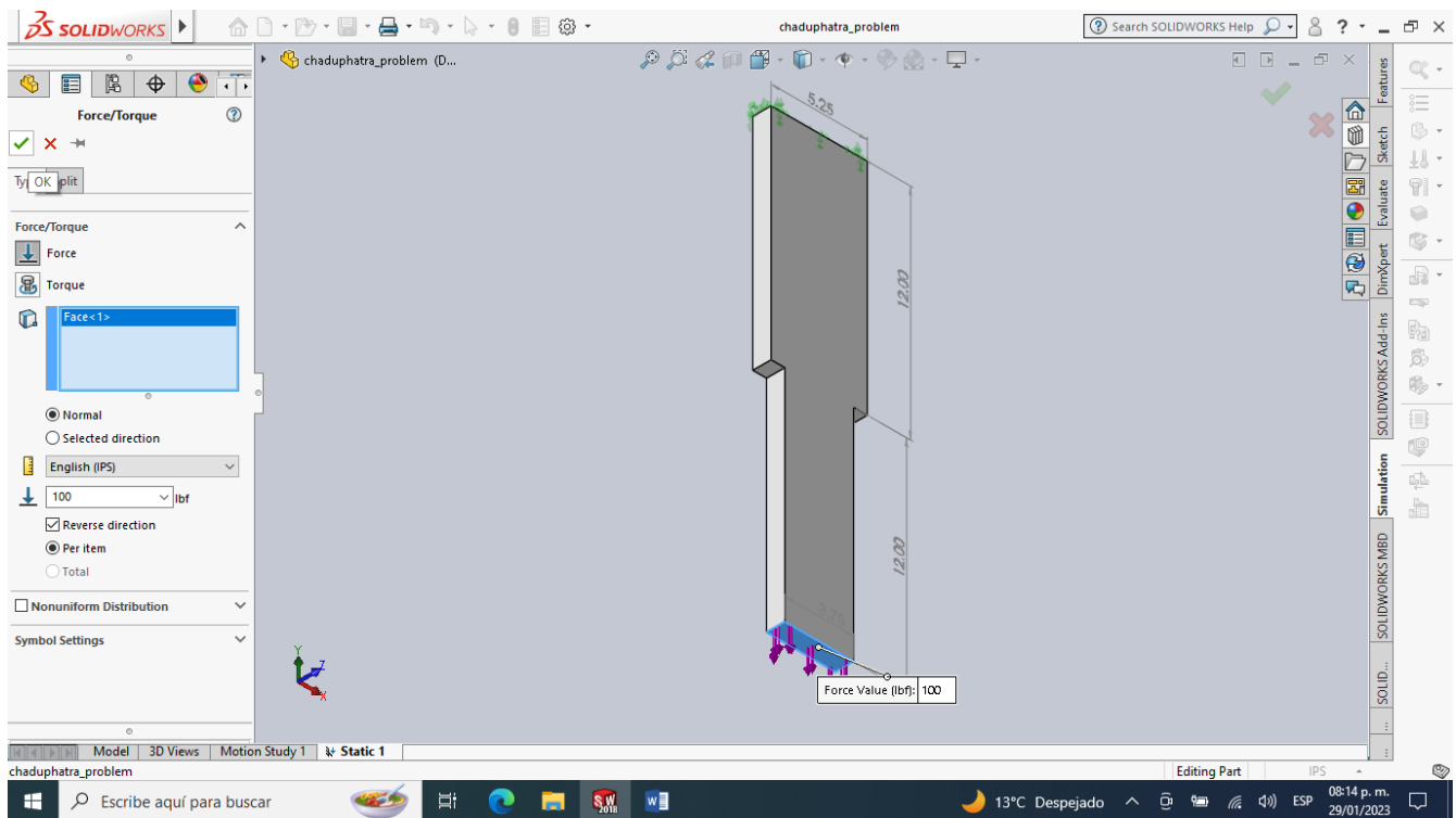
Figura 9. Seleccionar fuerza aplicada al sistema.
