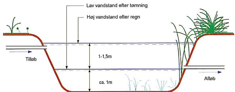
Figur 2. Principskitse af et vådt regnvandsbassin. Det nederste vandvolumen er bassinets permanente volumen og det øverste vandvolumen er bassinets magasin volumen.
