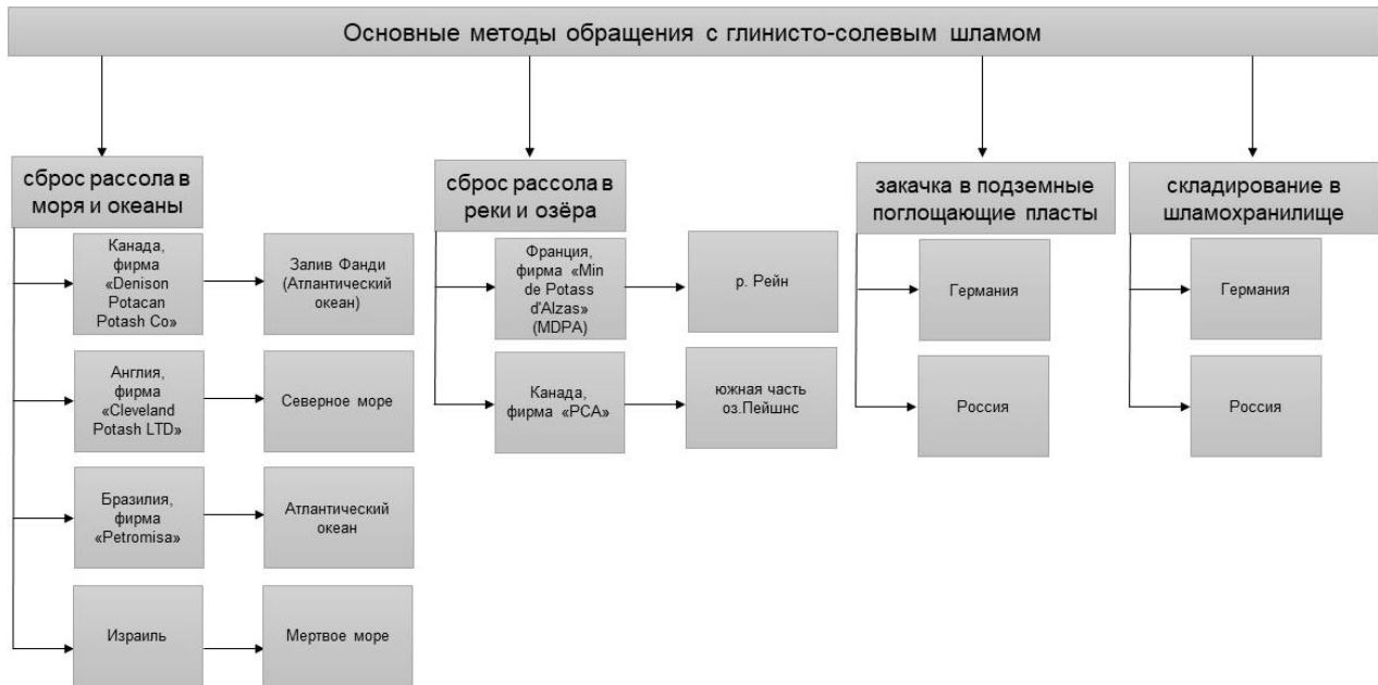
Рис. 4. Управление глинисто-солевым шламом Fig. 4. Management of clay-salt slurry
