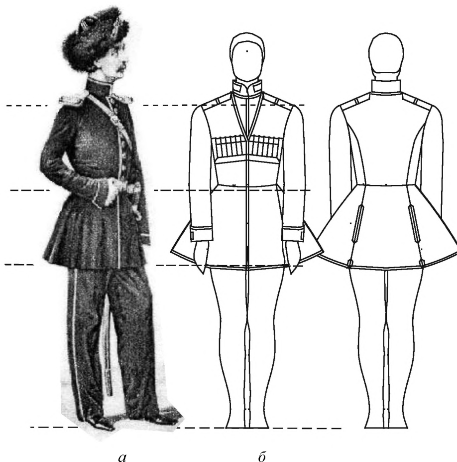
Рис. 2. а) обер-офицер Эриванского карабинерного полка ОККК (1848-1850 гг.); б) эскиз и чертеж конструкции экспоната КГИАМЗ (КМ.1639.Т-5)
