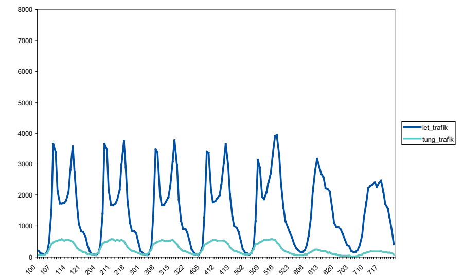
Figur: Trafikken ved Skanderborg fordelt på ugedage. Trafikken har klare myldretider for pendling i morgen og eftermiddagstimerne på hverdage, mens weekendtrafikken har et andet mønster med en top midt på dagen. Den tunge trafik udgør en stor andel på hverdage, men er langt lavere i weekenden.
