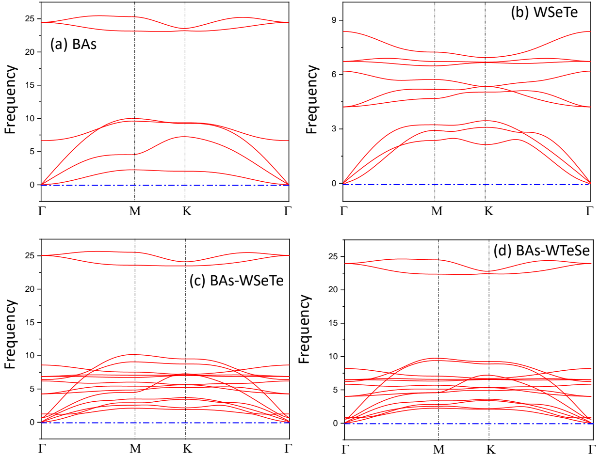
Figure 2. The phonon spectra of the (a) BAs, (b) WSeTe, (c) BAs-WSeTe, and (d) BAs-WTeSe heterostructures.
