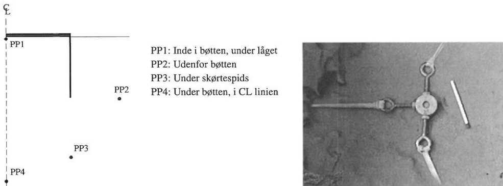
Figur 2 a) Principskitse af poretrykstransducernes placering b) Fiksering af poretrykstransducer, efter Leth og Mikkelsen (1998).
