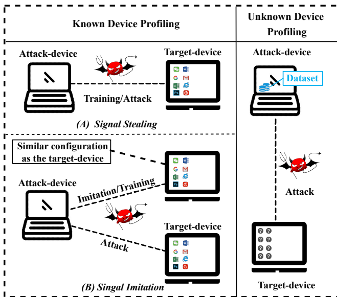
Fig. 4. Attack scenarios.
