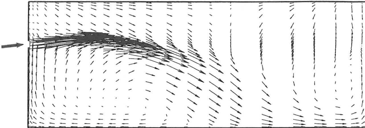
Figur 4.18. Beregning af en kold luftstråles forløb. Der indblæses 375 \text{ m}^3/\text{h} ved en hastighed på 1,9 \text{ m/s} og en undertemperatur på 10 \text{ }^\circ\text{C} . Figuren viser et snit midt for indblæsningen.
