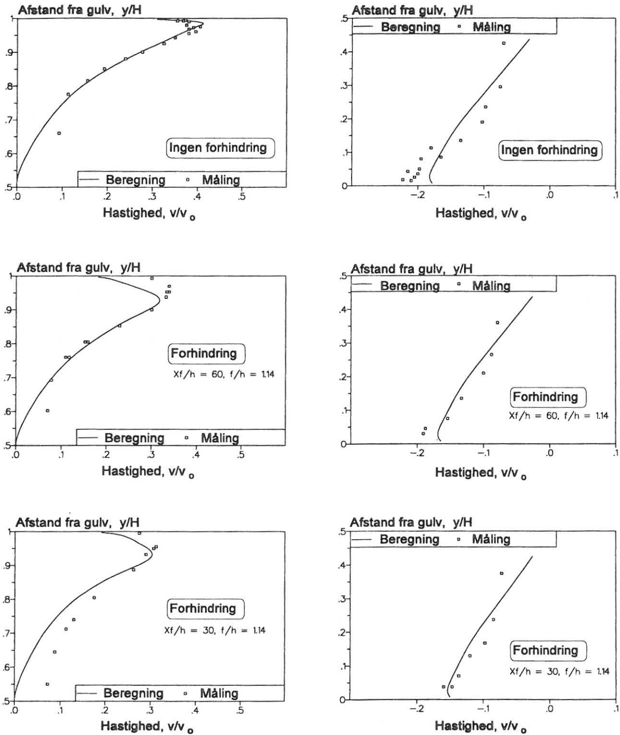
Figur 4.11. Sammenligning mellem computersimuleringer og laboratiormålinger af hastighedsprofiler, hvor luftstrålen har passeret en forhindring. Til venstre vises forholdene under loftet i afstanden 1,7 gange H fra indblæsningen og til højre forholdene i opholdszonen i afstanden 2,1 gange H fra indblæsningen.
