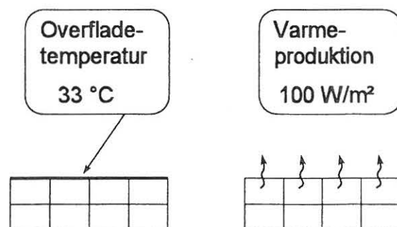
Figur 3.4. En varmekilde kan specificeres ved at angive en given overfladetemperatur eller ved at angive en kendt varmeproduktion pr. \text{m}^2 .
