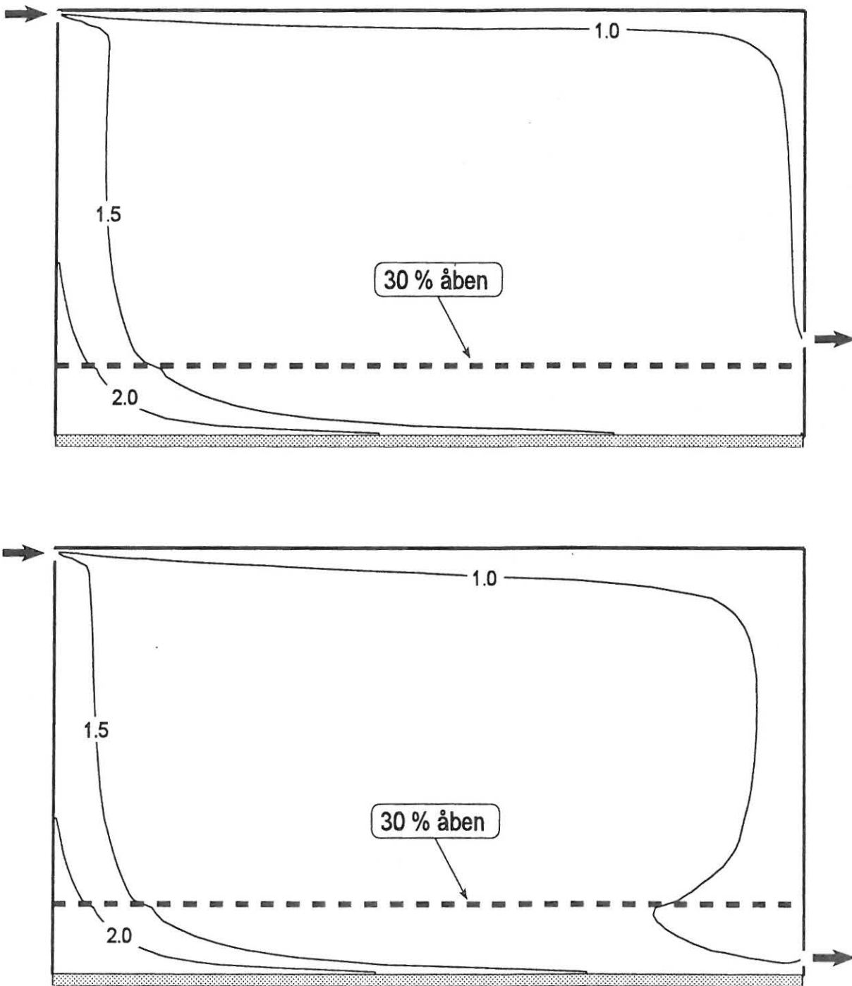
Figur 4.9. Beregnede forureningskoncentrationer i stalden ved udsugning over spaltegulvet (øverst) og udsugning under spaltegulvet (nederst). Kurverne viser koncentrationen i forhold til udsugningskoncentrationen. Det er forudsat, at forureningen frigives under spaltegulvet, og spaltegulvets åbningsgrad er 30 %.
