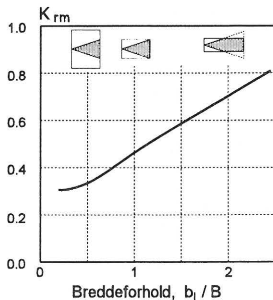
Figur 2.10. For en rund vægstråle afhænger K_{rm} af forholdet mellem strålens bredde b_L og området strålen skal dække B . Øverst i diagrammet illustreres bredderforholdet med skitser af en stråle, der blæses ind i rum af forskellig bredde.
