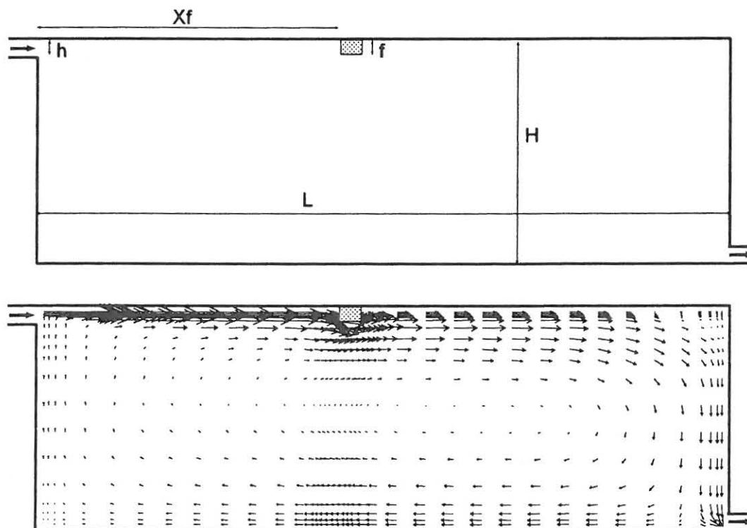
Figur 4.10. Forsøgsopstilling med en spalteindblæsning øverst til venstre, udsugning nederst til højre og en forhindring monteret under loftet. Indblæsningsspalten har højden h , forhindringen har tykkelsen f og sidder i afstanden Xf fra indblæsningen. Simuleringen viser, at luftstrålen fortsætter langs loftet efter at have passeret forhindringen.
