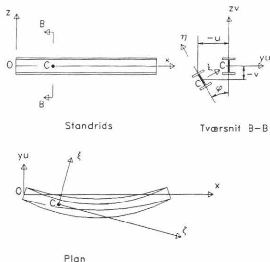
Figur 3. Bjælkens deformationer
