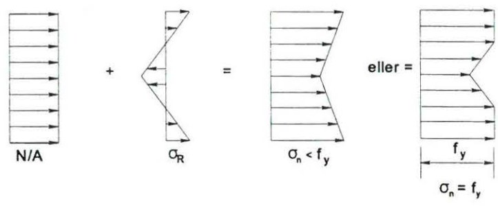
Figur 12. Eksempler på virkningen af egenspændingsfordelinger
