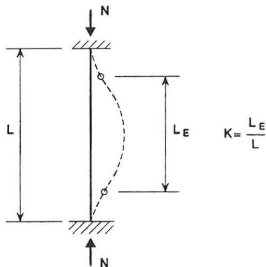
Figur 2. Fri søjlelængde.
