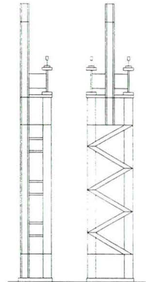
Figur 8. Sammensat søjle med varierende tværsnit
