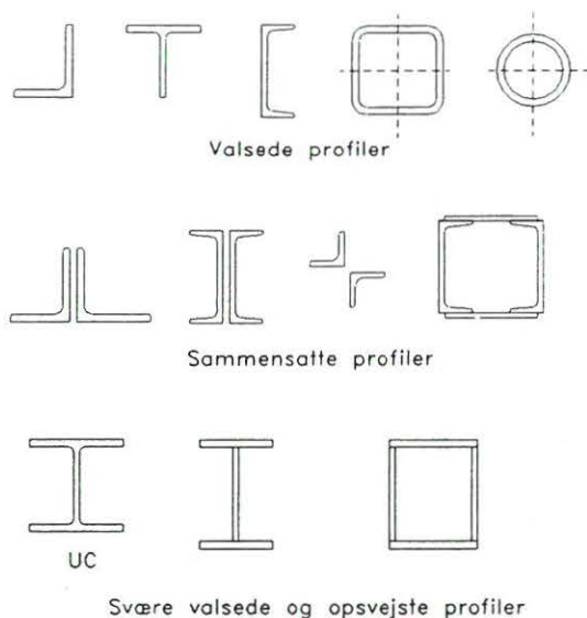
Figur 4. Tværsnit af trækstænger
