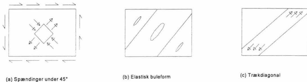
Figur 7 Forskydningsfoldning
