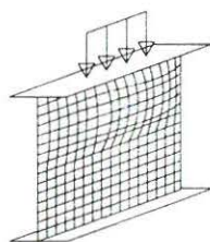
(c) Kropplade med koncentreret last
