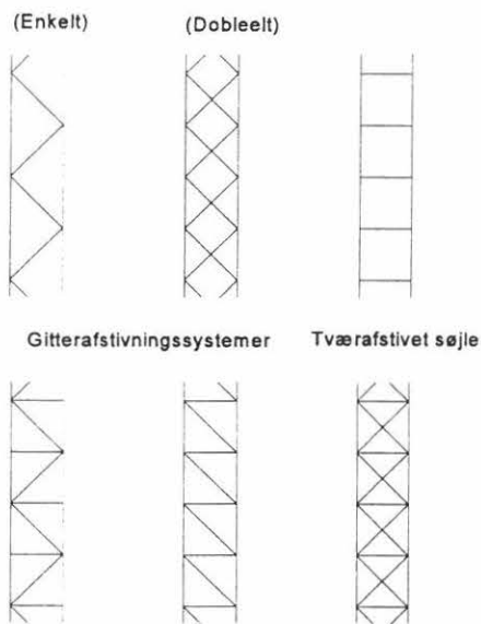
Kombinationer af gitter- og tværafstivninger
