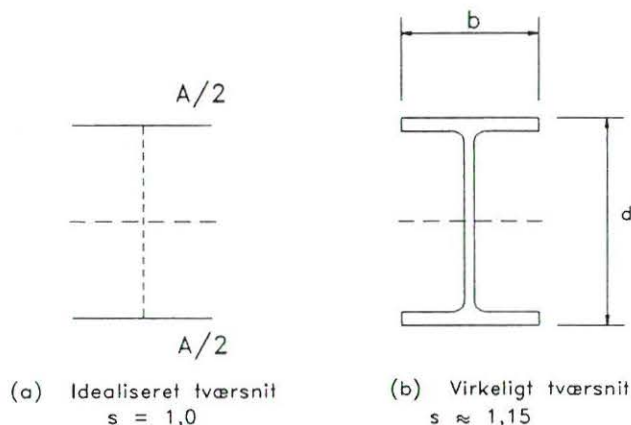
Figur 7. I-tværsnit
