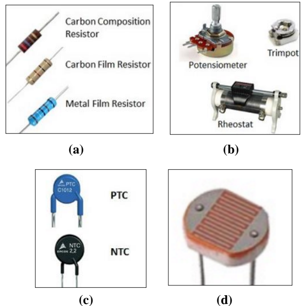
Gambar 2. Bentuk dan Jenis Resistor: (a) Fixed, (b) Variable, (c) Thermal, (d) Light Dependent
